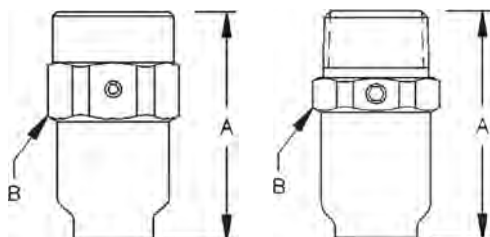
60° / 90° / 120° Femelle
